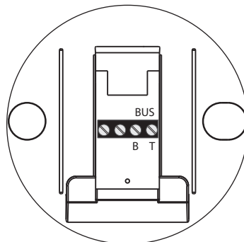
Płytki zaciskowa panelu zdalnego sterowania
