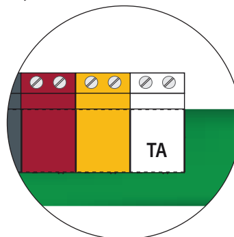
Płytki zaciskowa Bus modułu
