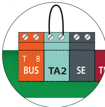
Płytki zaciskowa Bus kotła
